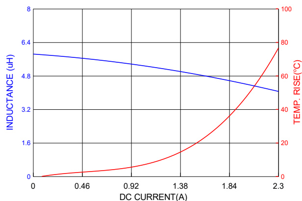
PIC0315H5R6MF
