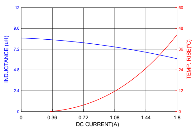
PIC0315H8R2MF
