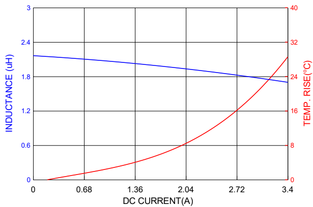
PIC0312H2R2MF
