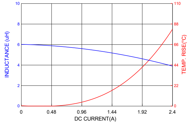
PIC0312H5R6MF
