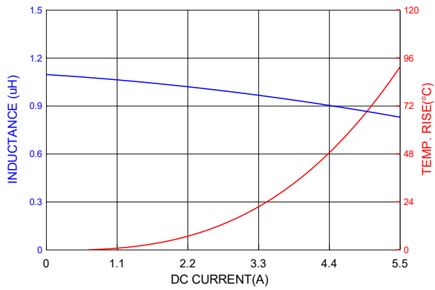
PIC0312H1R0MF
