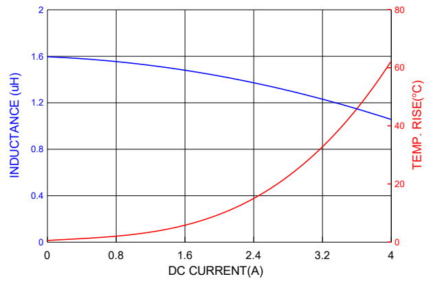
PIC0312H1R5MF
