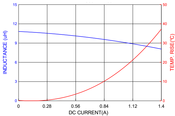
PIC0312H100MF
