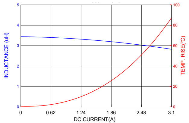
PIC0312H3R3MF
