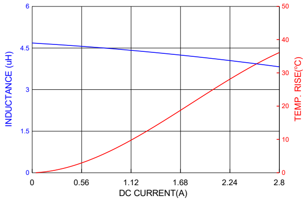
PIC0312H4R7MF
