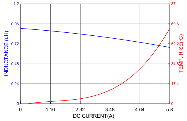
PIC0312HR82MF
