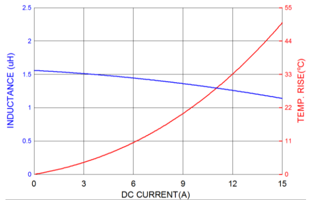
PIVQ0603S1R5MN
