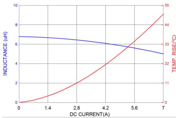
PIVQ0603S6R8MN
