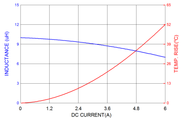
PIVQ0603S100MN
