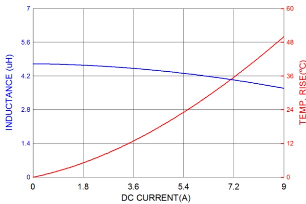
PIVQ0603S4R7MN
