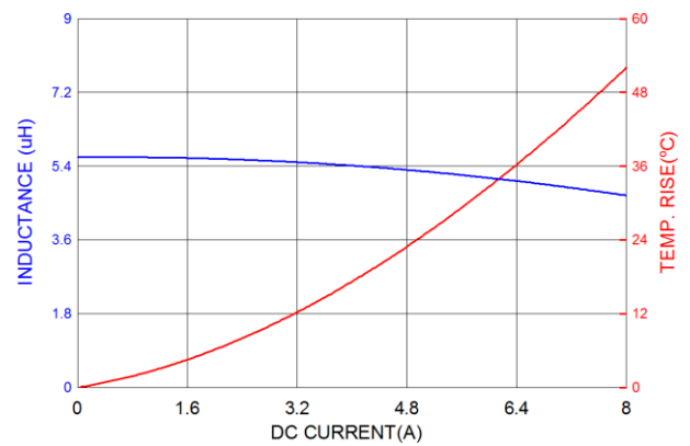
PIVQ0603S5R6MN
