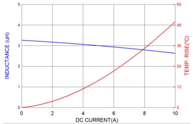
PIVQ0603S3R3MN
