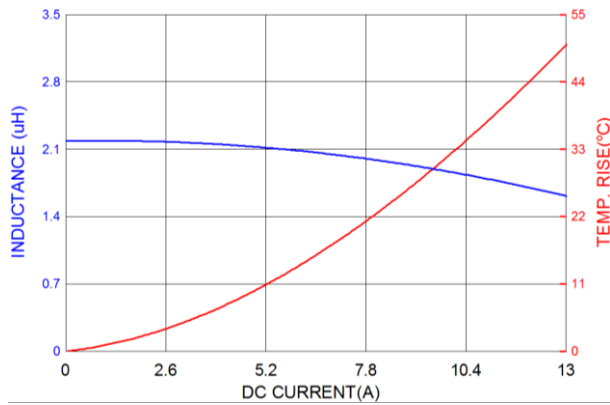
PIVQ0603S2R2MN
