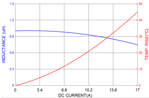
PIVQ0603S1R0MN
