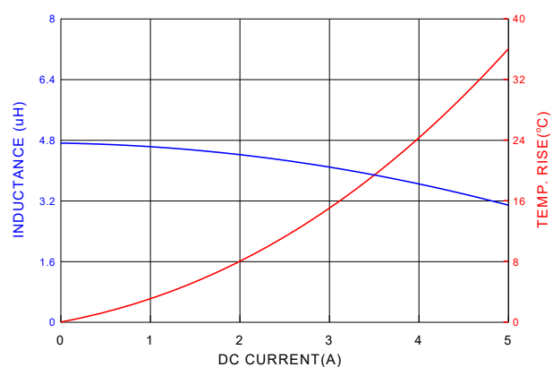
PIFQ0402LR4R7MN
