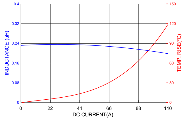
PICQ1205HPR22MF
