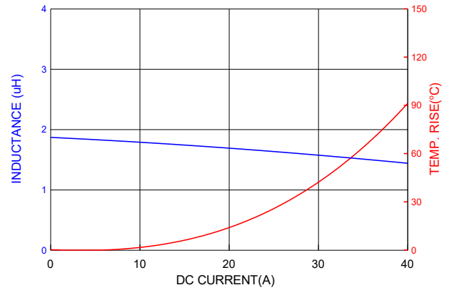
PICQ1205HP1R8MF
