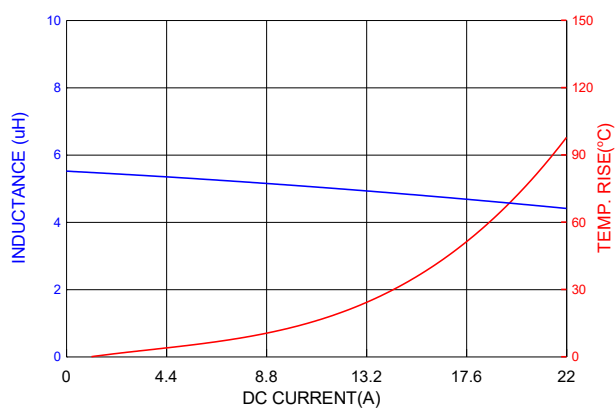
PICQ1205HP5R6MF
