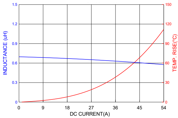
PICQ1205HPR68MF
