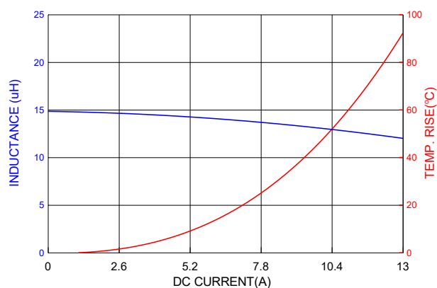
PICQ1205HP150MF
