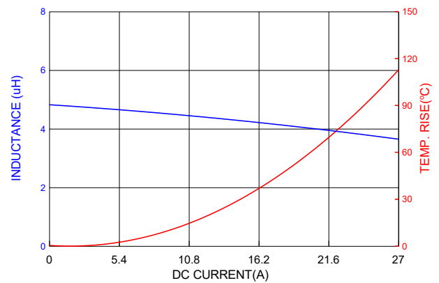
PICQ1205HP4R7MF
