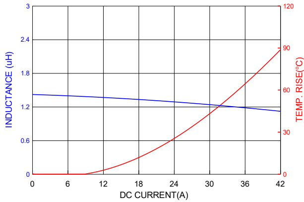
PICQ1205HP1R5MF
