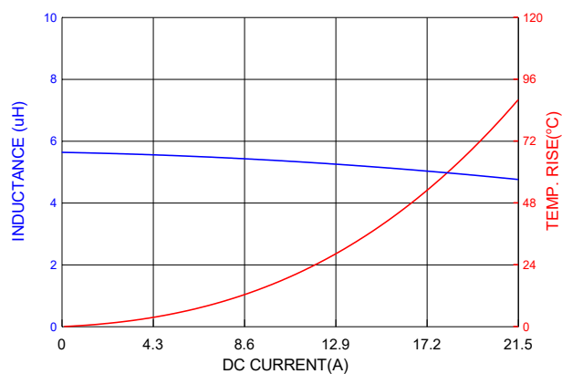
PICQ1205HP6R0MF
