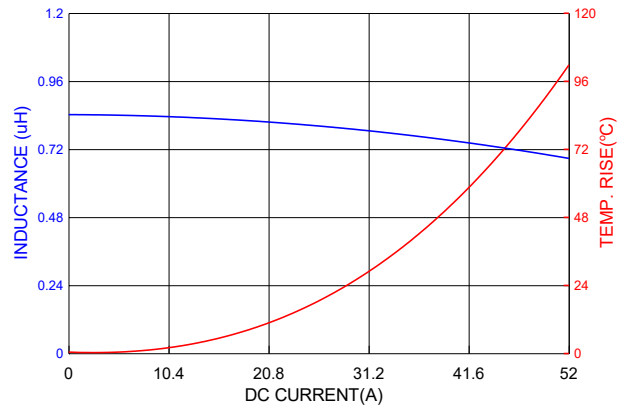
PICQ1205HPR82MF
