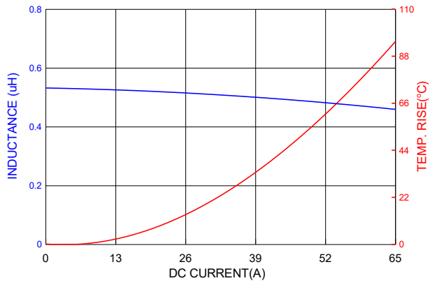
PICQ1205HPR50MF
