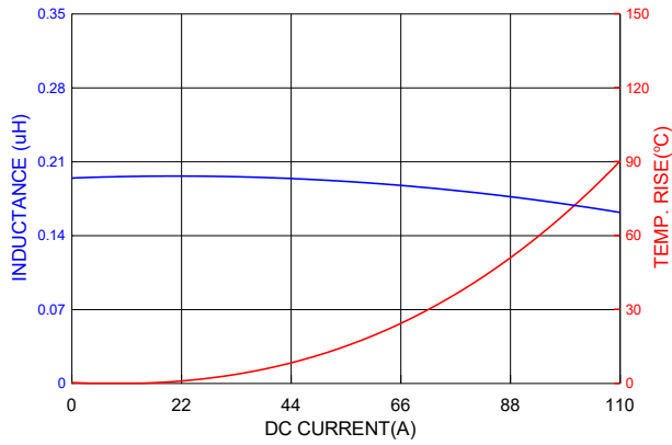
PICQ1205HPR20MF
