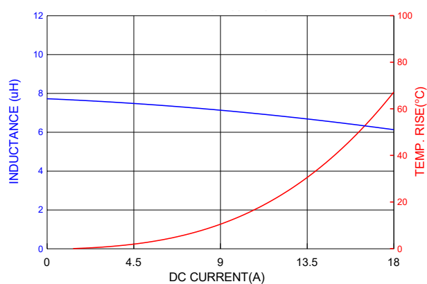
PICQ1205HP8R2MF
