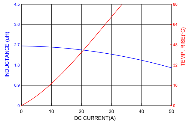
PICQ1205HP2R7MF
