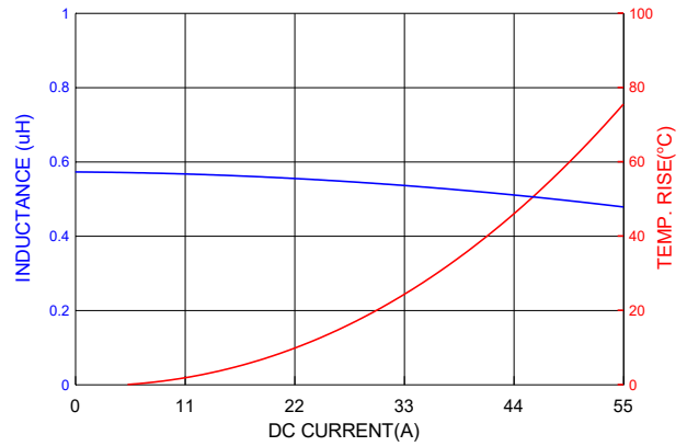
PICQ1205HPR56MF
