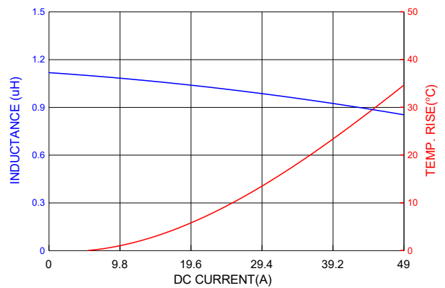
PICQ1205HP1R2MF
