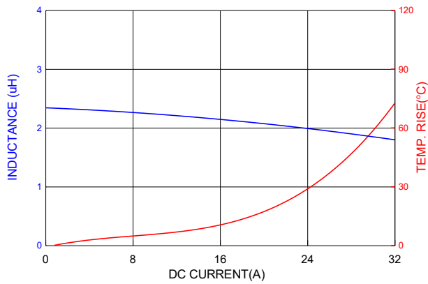
PICQ1205HP2R2MF
