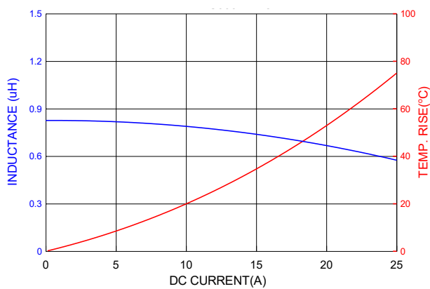
PICQ0604HR82MF
