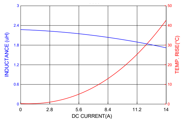
PICQ0604H2R2MF
