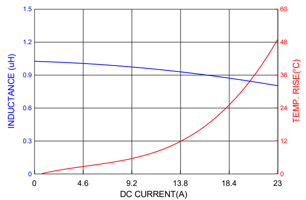
PICQ0604H1R0MF
