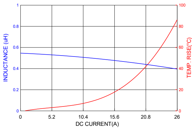
PICQ0604HR56MF
