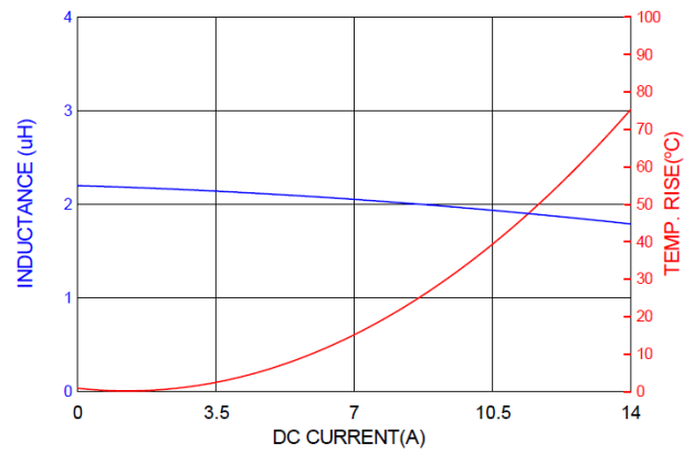
PICQ0603H2R2MF
