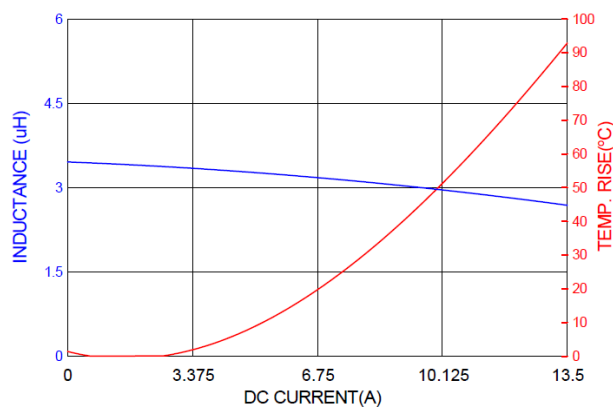
PICQ0603H3R3MF
