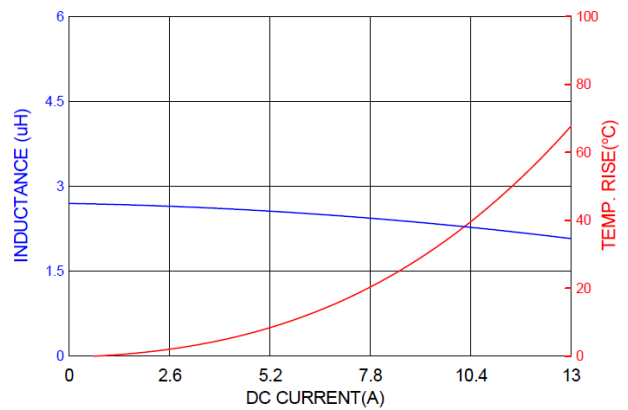
PICQ0603H2R7MF
