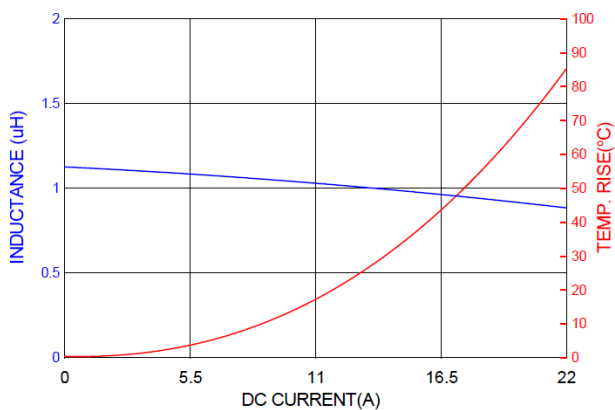
PICQ0603H1R0MF
