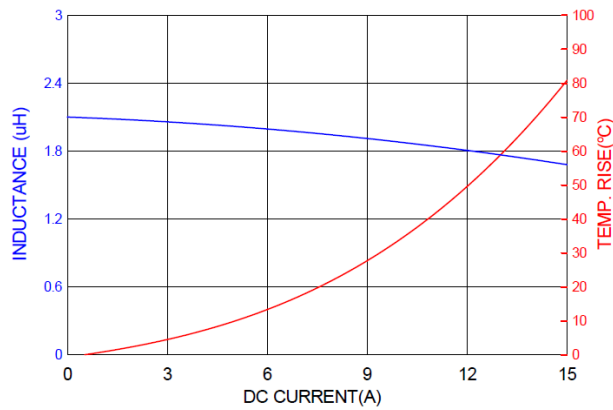
PICQ0603H2R0MF
