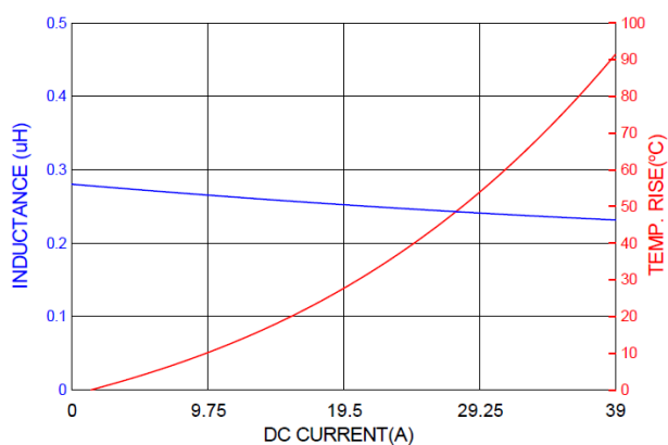
PICQ0603HR25MF
