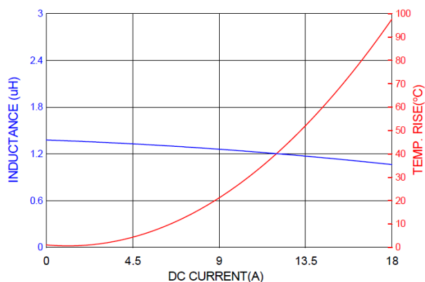
PICQ0603H1R5MF
