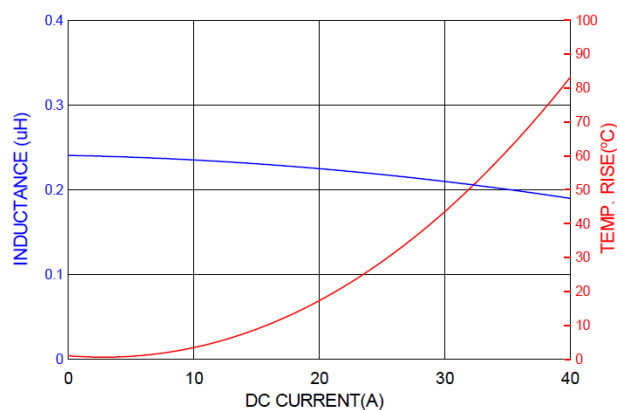
PICQ0603HR22YF
