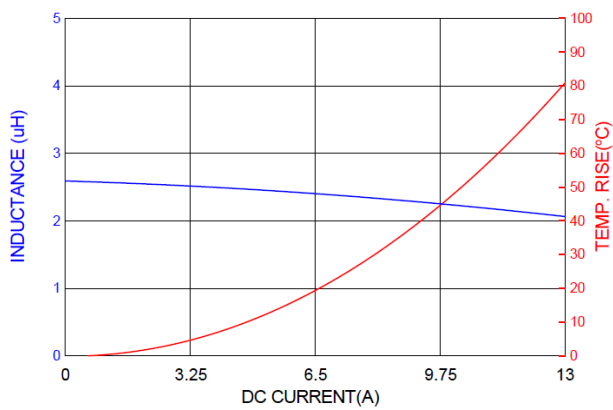
PICQ0603H2R5MF
