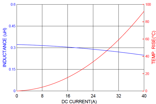
PICQ0603HR30MF
