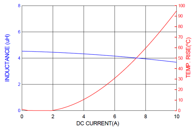
PICQ0603H4R7MF
