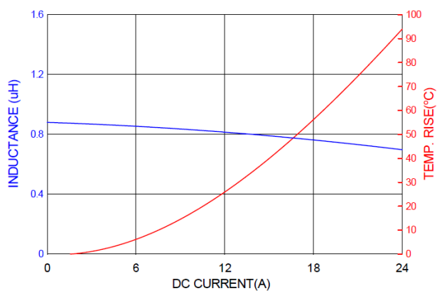
PICQ0603HR82MF
