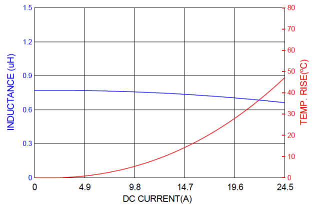
PICQ0603HR75MF
