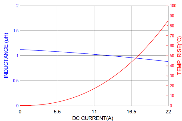
PICQ0603HR90MF
