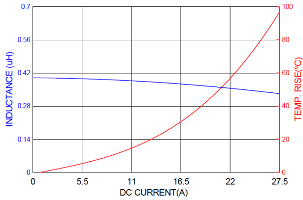
PICQ0603HR40MF
