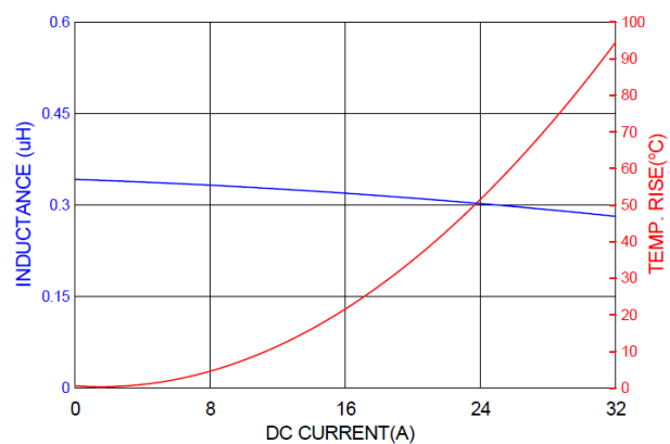
PICQ0603HR36MF
