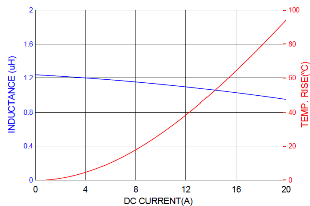
PICQ0603H1R2MF
