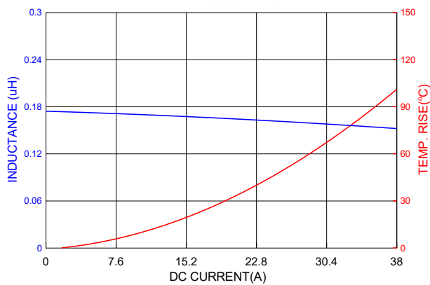
PICQ0602HR16YF
