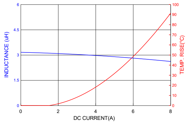
PICQ0602H3R3MF
