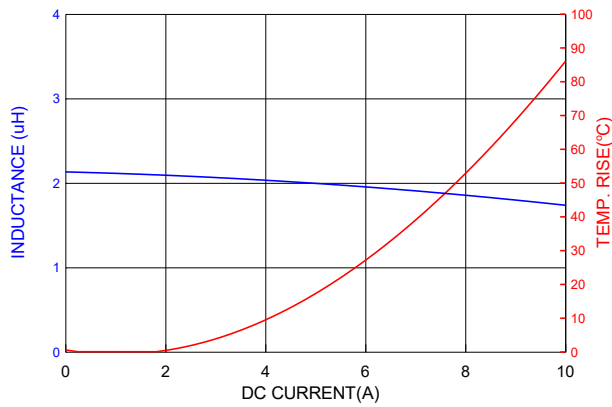
PICQ0602H2R2MF
