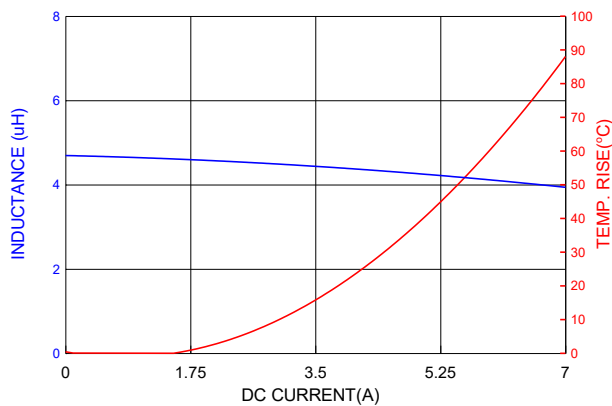
PICQ0602H4R7MF
