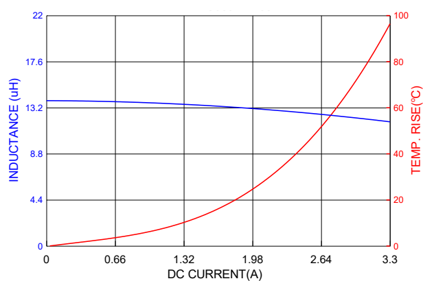
PICQ0602H150MF
