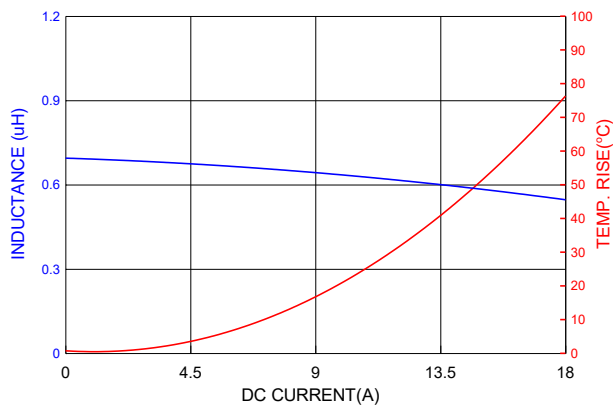
PICQ0602HR68MF
