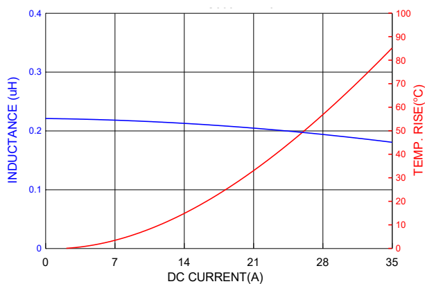
PICQ0602HR20YF
