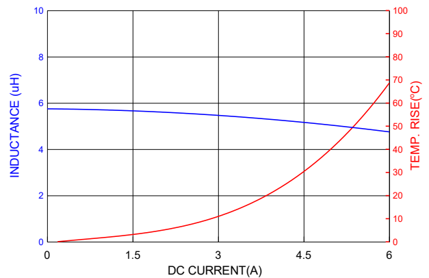
PICQ0602H5R6MF
