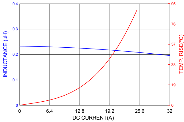
PICQ0602HR24MF
