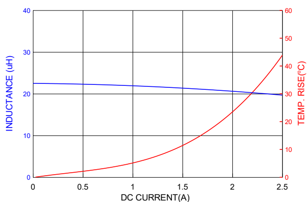
PICQ0602H220MF
