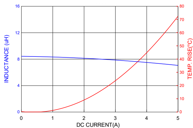
PICQ0602H8R2MF
