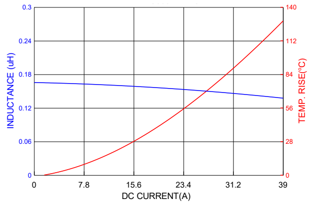
PICQ0602HR15YF
