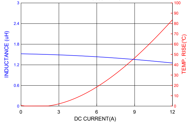
PICQ0602H1R5MF
