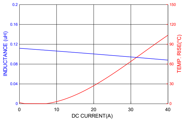
PICQ0602HR10YF
