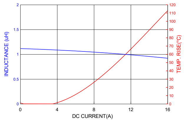
PICQ0602H1R0MF
