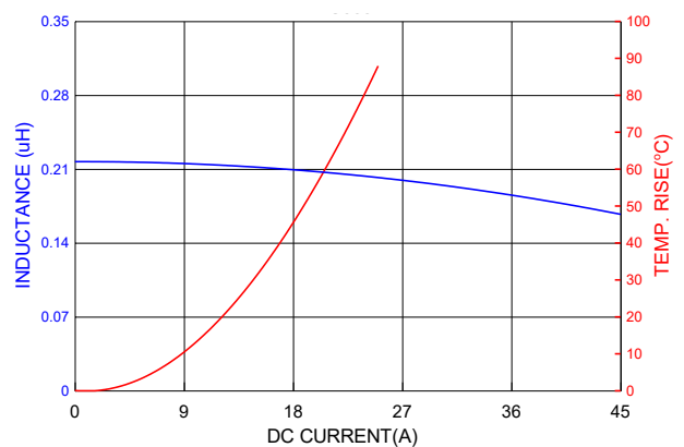
PICQ0602HR22YF
