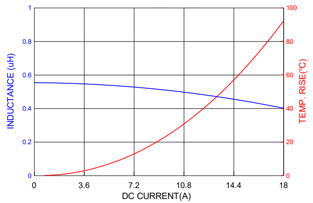
PICQ0602HR56MF
