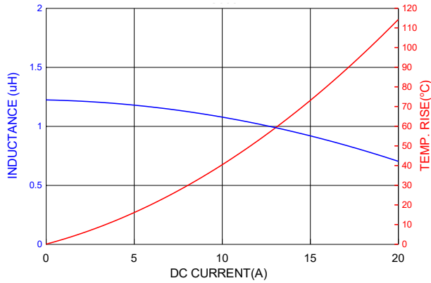
PICQ0602H1R2MF
