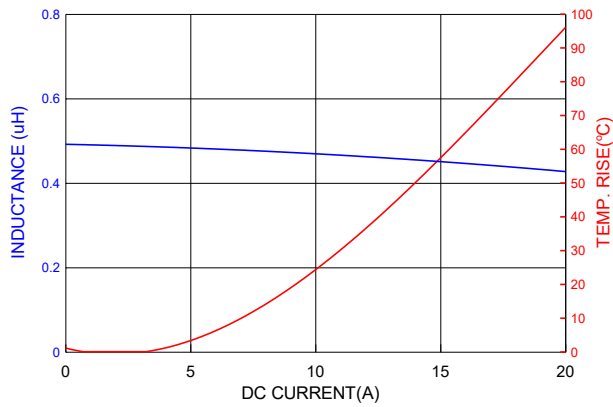
PICQ0602HR47MF
