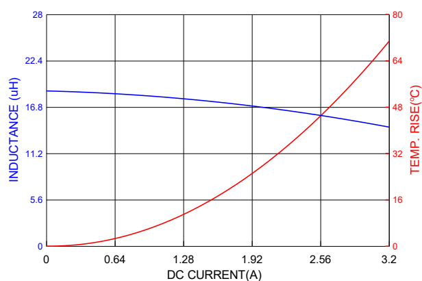
PICQ0503H180MF
