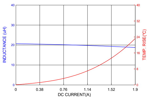
PICQ0503H220MF
