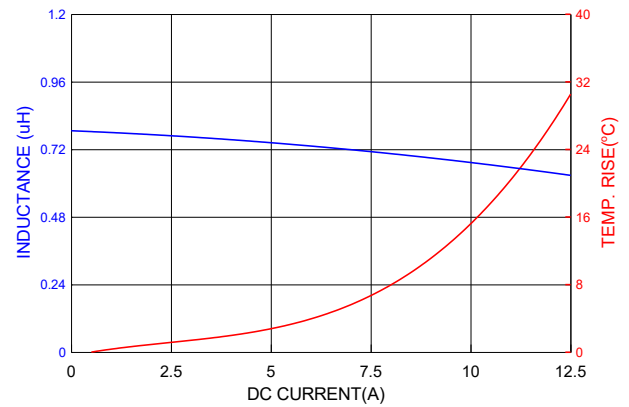
PICQ0503HR82MF
