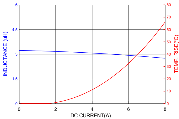
PICQ0503H3R3MF
