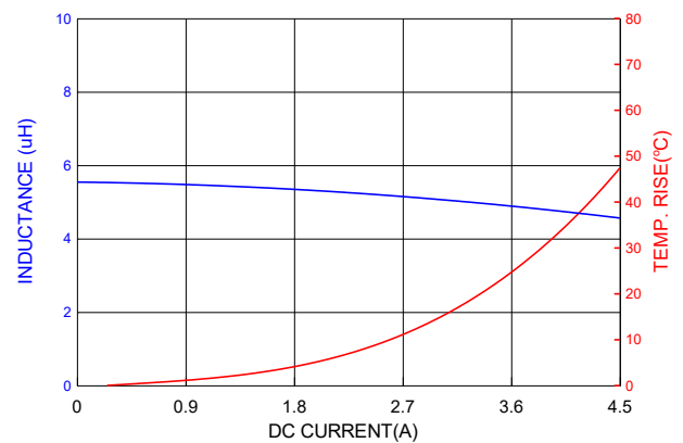
PICQ0503H5R6MF
