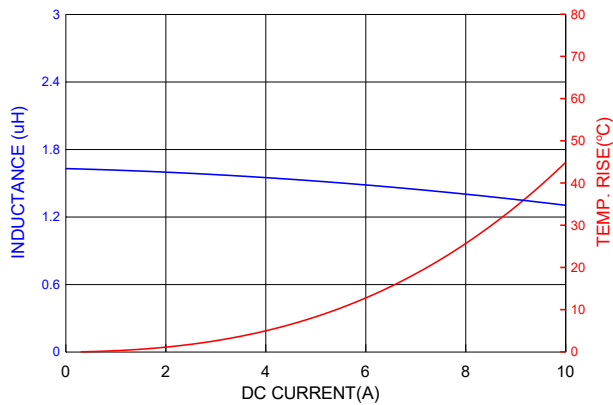
PICQ0503H1R5MF
