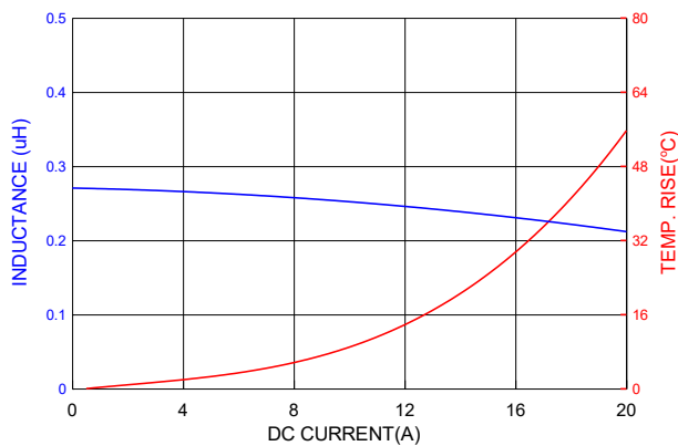
PICQ0503HR25MF
