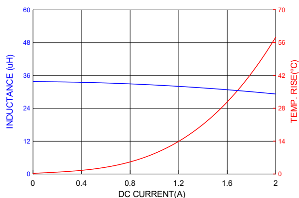
PICQ0503H330MF
