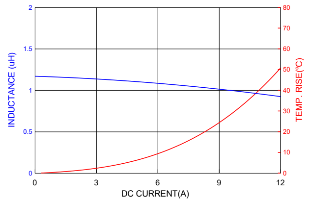
PICQ0503H1R2MF
