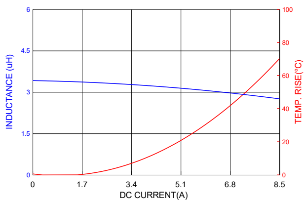
PICQ0503HP3R3MF
