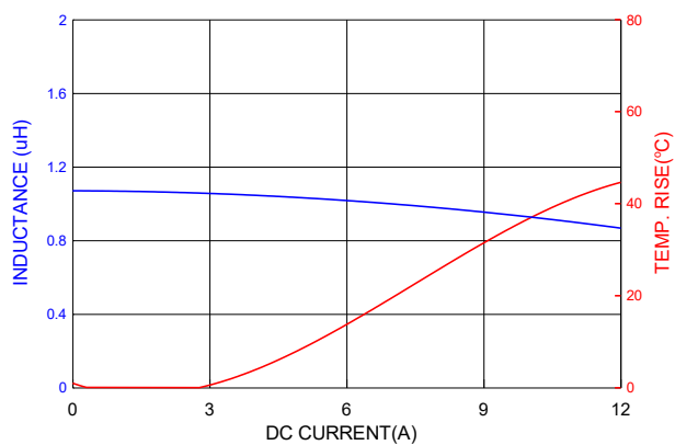
PICQ0503HP1R0MF
