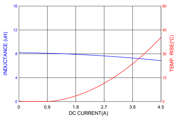
PICQ0503HP8R2MF
