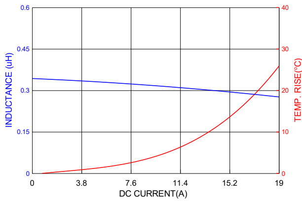
PICQ0503HPR33MF
