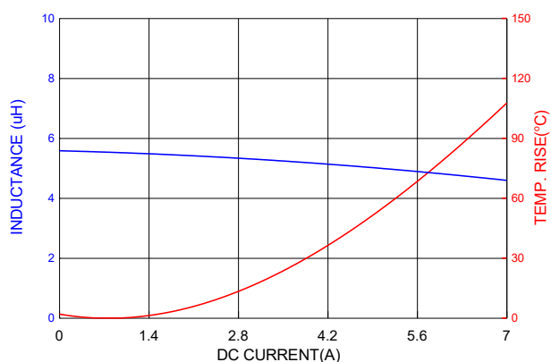
PICQ0503HP5R6MF
