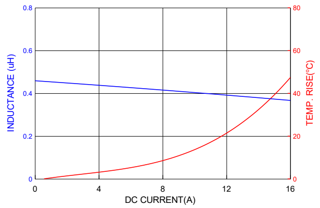
PICQ0503HPR47MF
