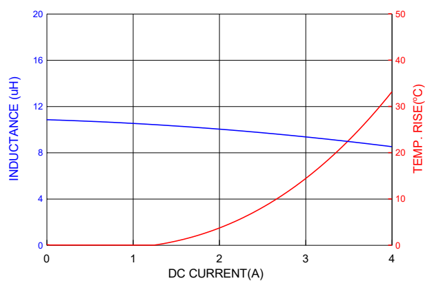
PICQ0503HP100MF
