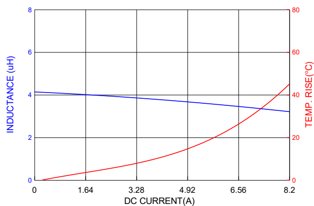
PICQ0503HP4R7MF
