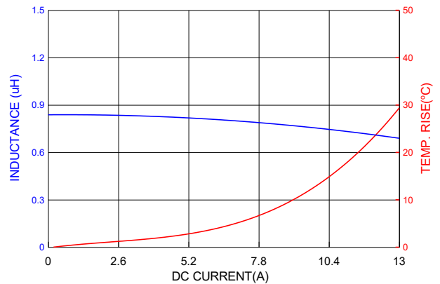
PICQ0503HPR82MF
