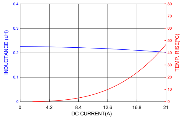
PICQ0503HPR22MF
