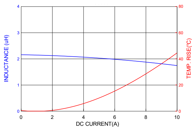
PICQ0503HP2R2MF
