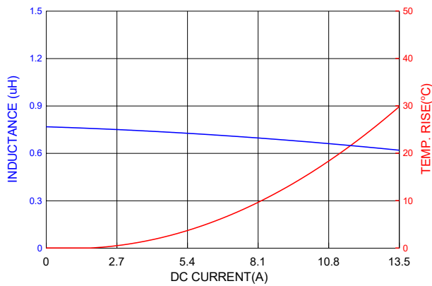
PICQ0503HPR68MF
