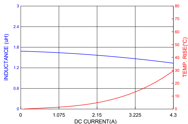
PICQ0412HP1R5MF
