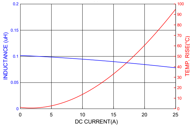
PICQ0412HPR10YF
