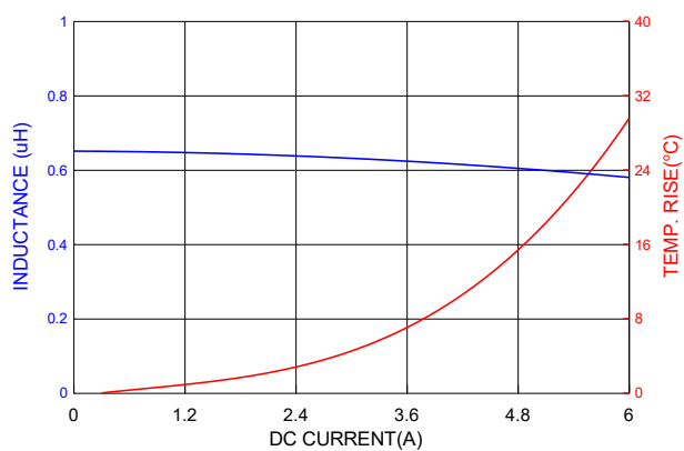
PICQ0412HPR68MF
