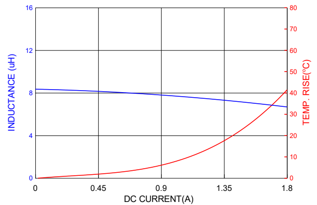
PICQ0412HP8R2MF
