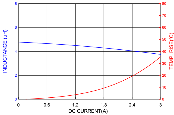
PICQ0412HP4R7MF
