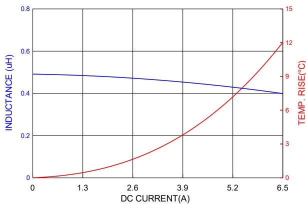
PICQ0412HPR47MF
