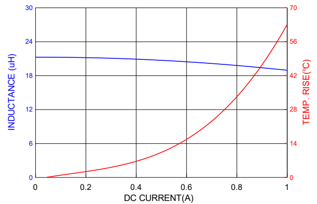
PICQ0412HP220MF
