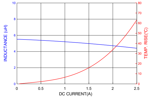
PICQ0412HP5R6MF
