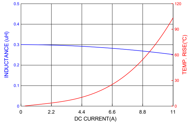
PICQ0412HPR22MF
