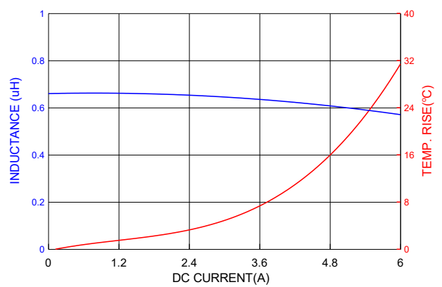
PICQ0412HPR60MF
