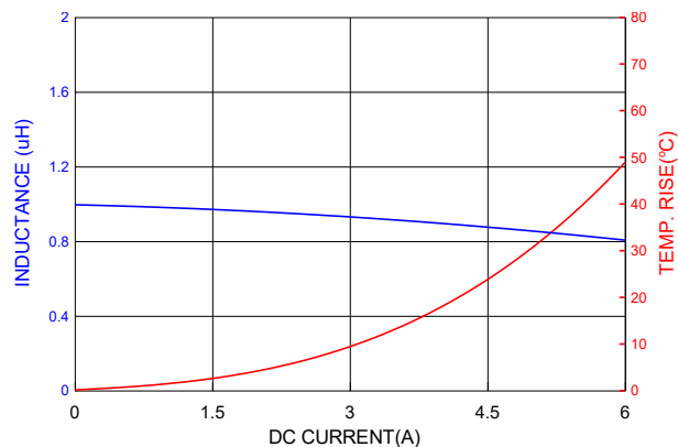
PICQ0412HP1R0MF
