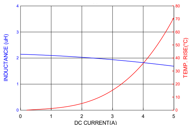
PICQ0412HP2R2MF
