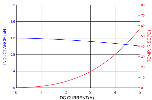
PICQ0412HP1R2MF
