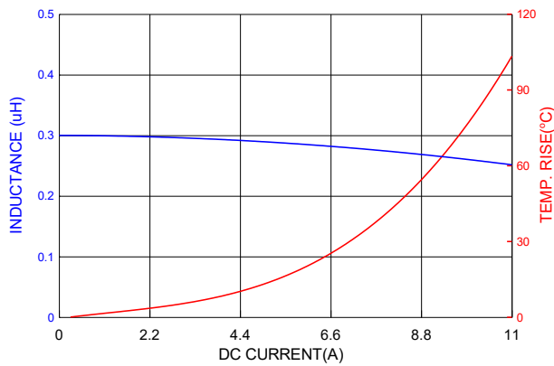
PICQ0412HPR33MF
