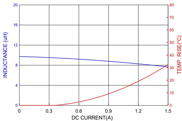
PICQ0412HP100MF
