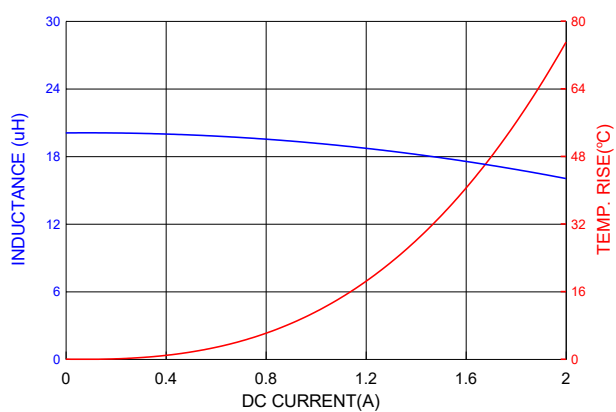
PICQ0402HP200MF
