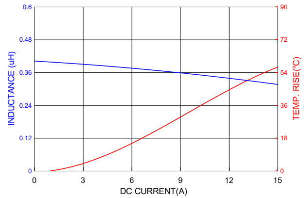
PICQ0402HPR33MF
