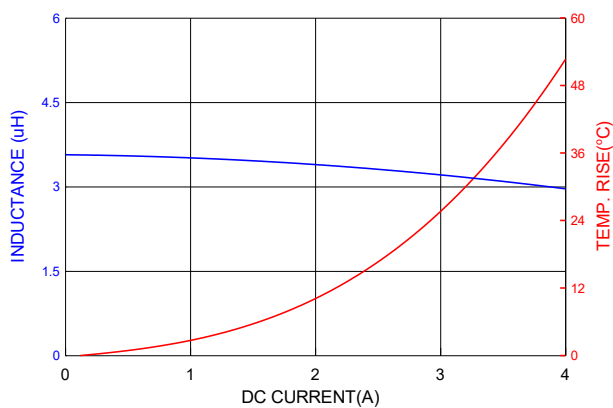
PICQ0402HP1R5MF
