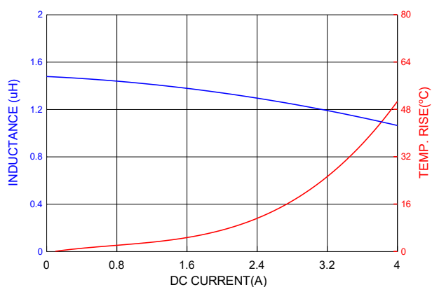
PICQ0318H1R5MF
