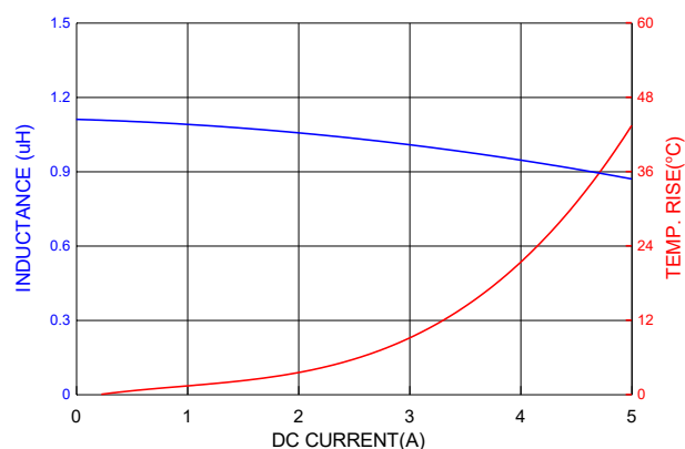
PICQ0318H1R0MF
