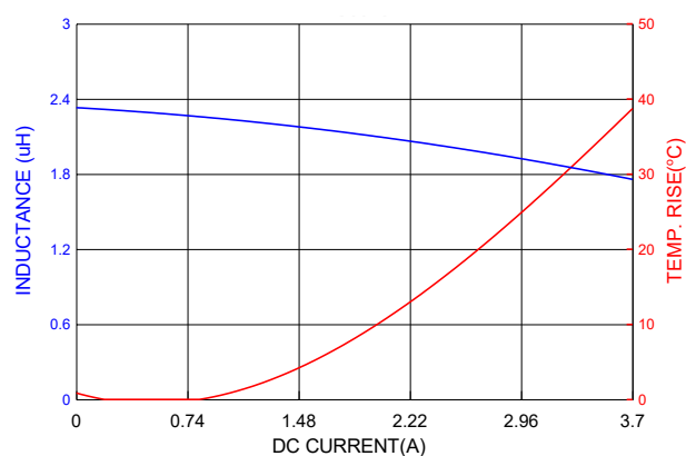
PICQ0318H2R2MF
