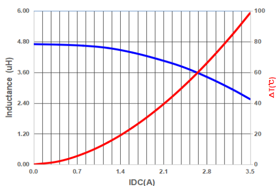
PIM252012A4R7M
