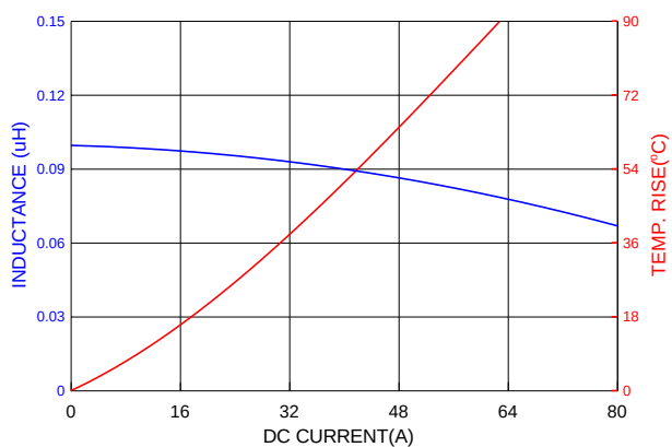
PIAQ0624SR10YN
