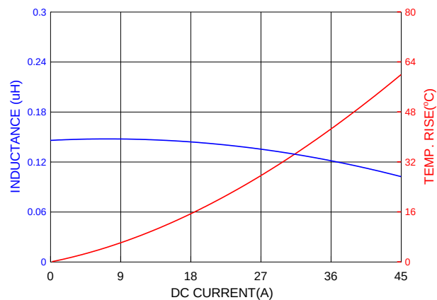
PIAQ0624SR15MN
