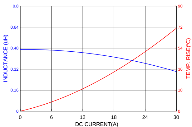
PIAQ0624SR47MN
