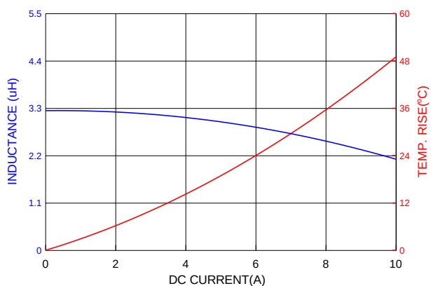
PIAQ0624S3R3MN
