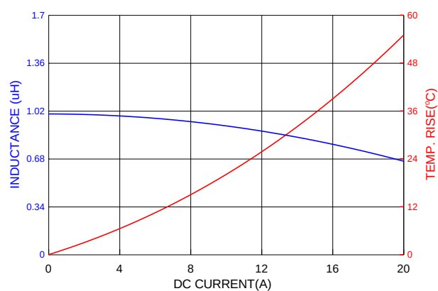
PIAQ0624S1R0MN
