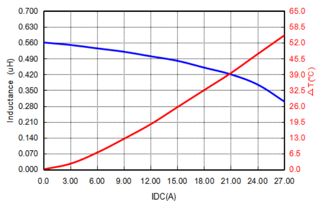
PIAQ0605SR56MN
