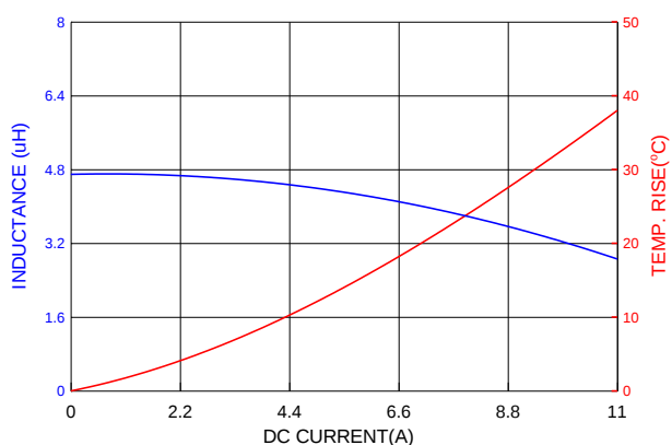
PIAQ0605S4R7MN
