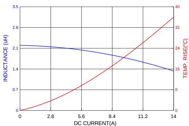
PIAQ0605S2R2MN
