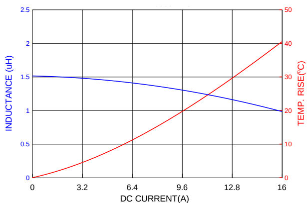
PIAQ0605S1R5MN
