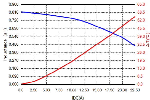
PIAQ0605SR82MN
