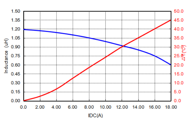
PIAQ0605S1R2MN
