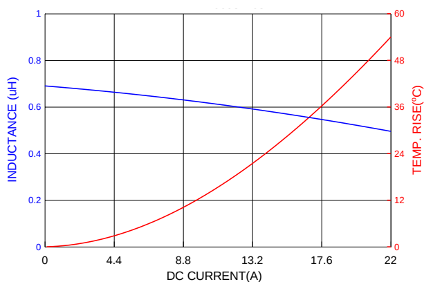
PIAQ0603SR68MN
