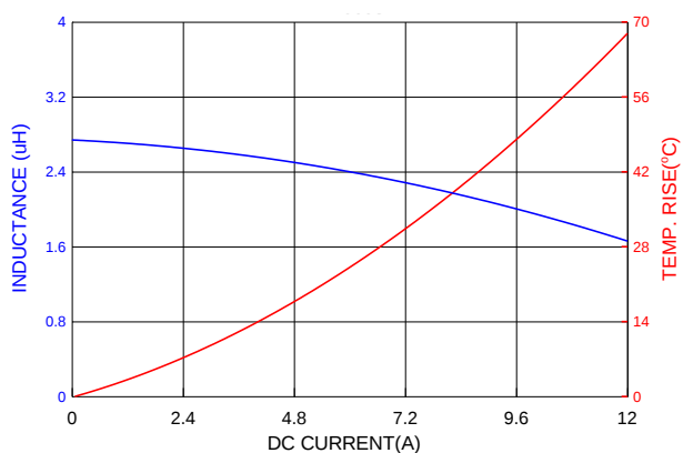
PIAQ0603S2R7MN
