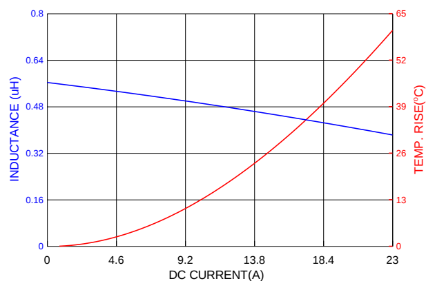
PIAQ0603SR56MN
