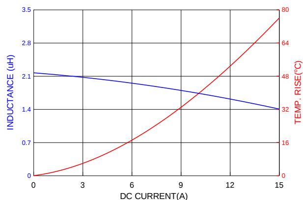
PIAQ0603S2R2MN
