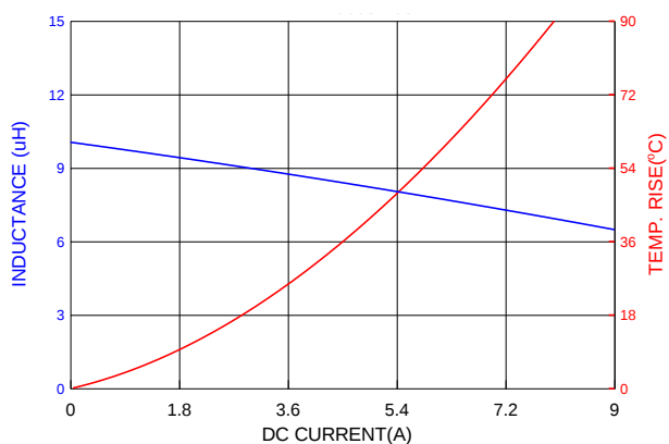
PIAQ0603S100MN
