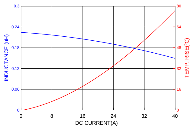
PIAQ0603SR22MN
