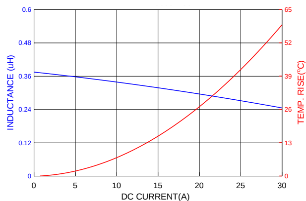
PIAQ0603SR36MN
