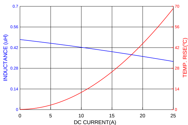
PIAQ0603SR47MN
