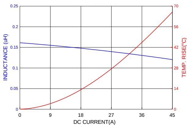
PIAQ0603SR15YN
