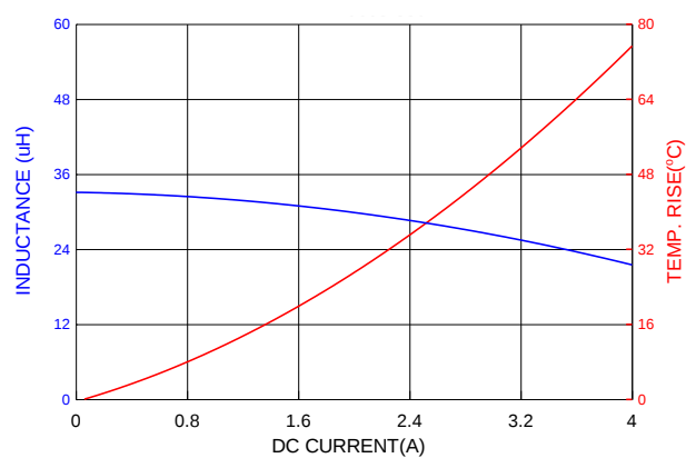
PIAQ0603S330MN
