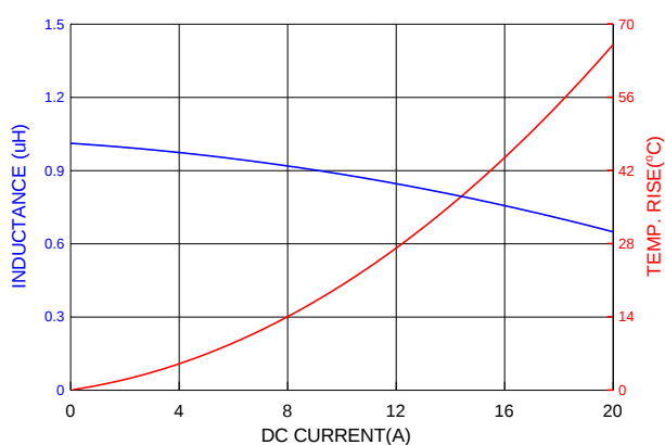
PIAQ0603S1R0MN
