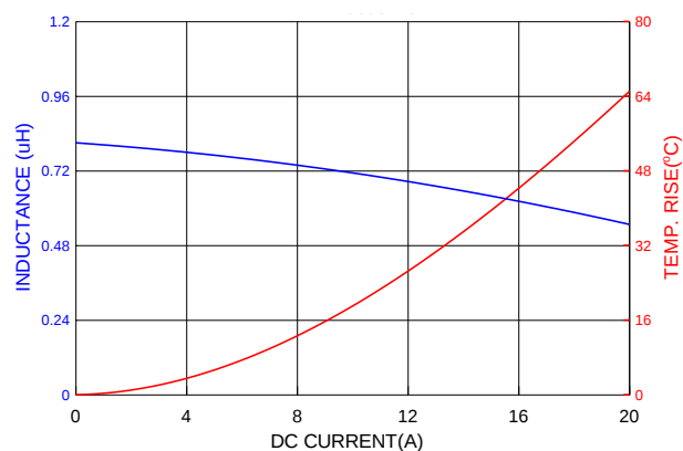
PIAQ0603SR82MN
