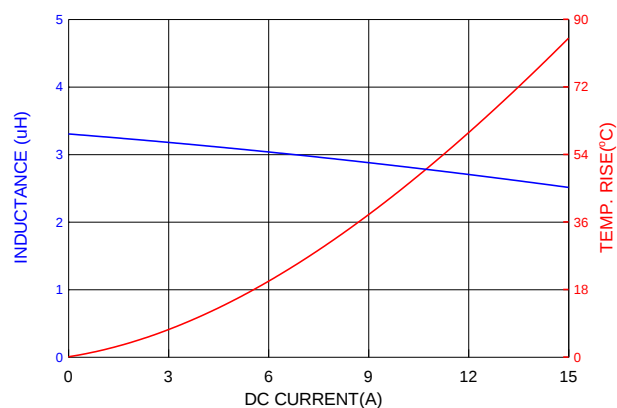
PIAQ0603S3R3MN
