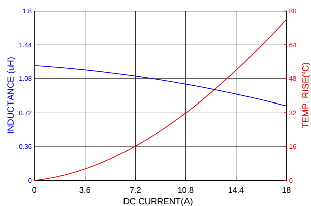
PIAQ0603S1R2MN
