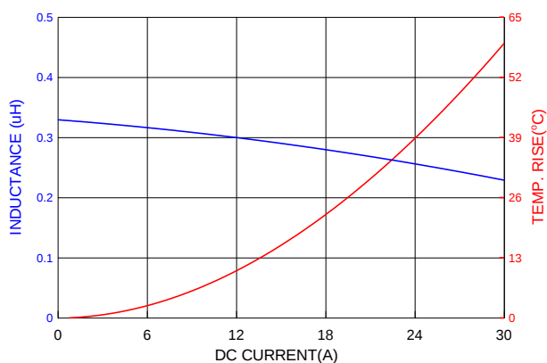
PIAQ0603SR33MN
