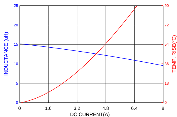
PIAQ0603S150MN
