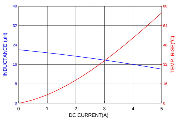
PIAQ0603S220MN
