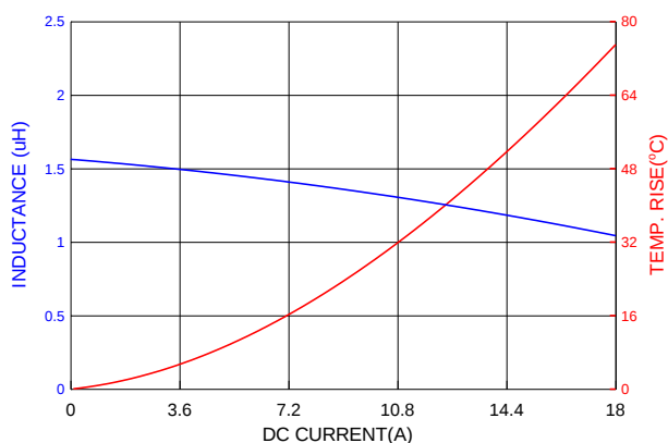
PIAQ0603S1R5MN
