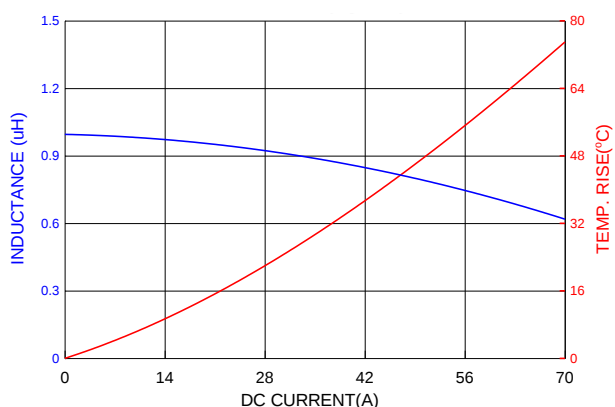
PIA1707SP1R0MN
