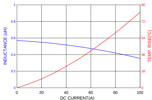
PIA1707SPR56MN
