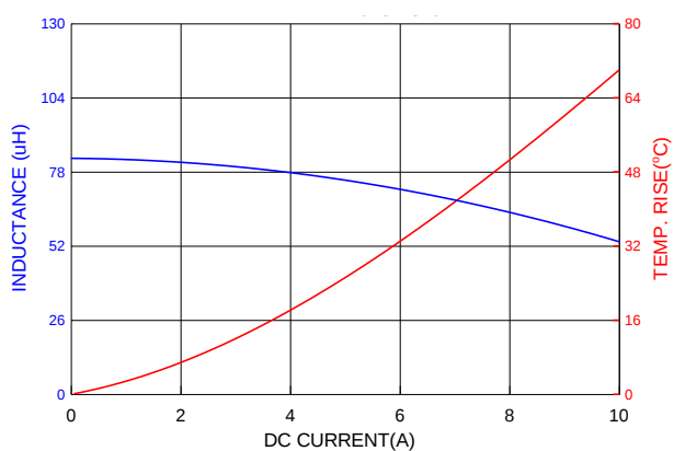
PIA1707SP820MN
