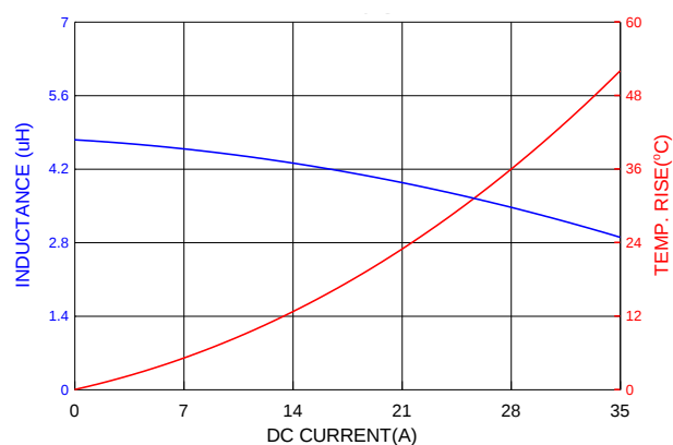
PIA1707SP4R7MN
