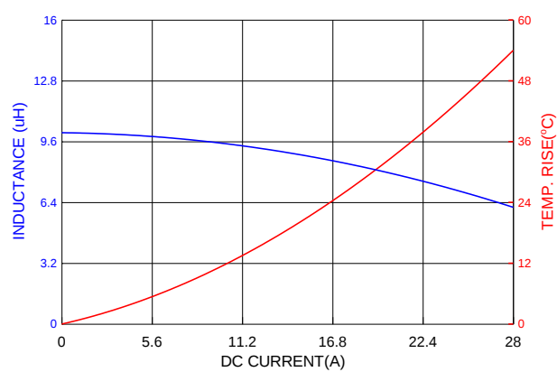
PIA1707SP100MN
