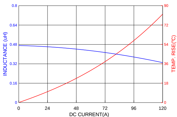
PIA1707SPR47MN
