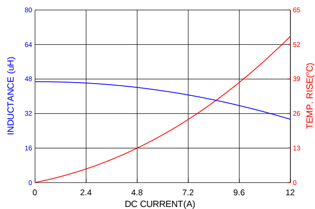
PIA1707SP470MN
