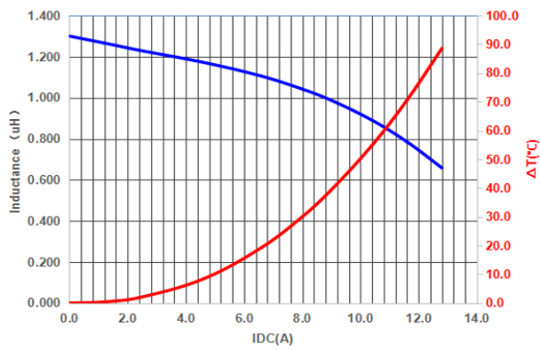
PIF0402A1R2MN
