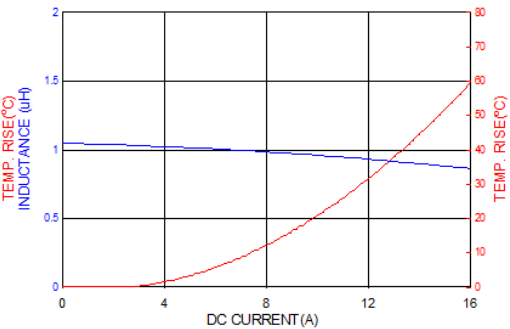
PICQ0624H1R0MF
