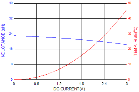
PICQ0624H220MF
