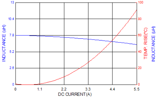
PICQ0624H8R2MF
