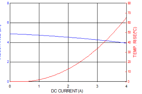
PICQ0612H4R7MF
