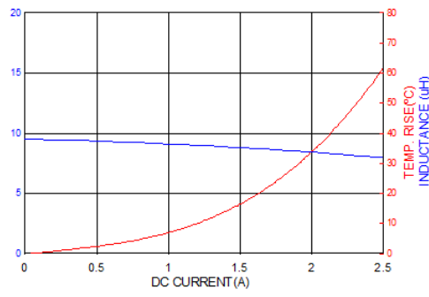
PICQ0612H100MF
