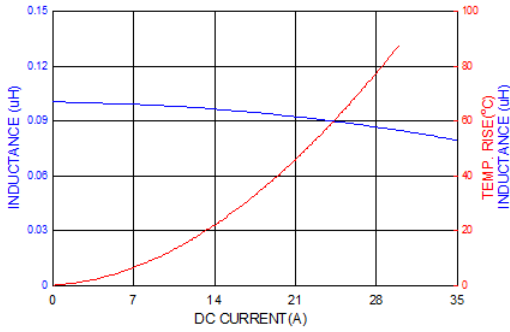
PICQ0612HR10YF
