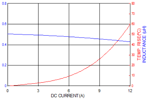
PICQ0612HR47MF
