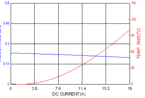
PICQ0612HR22YF
