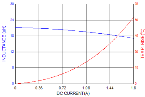
PICQ0612H220MF
