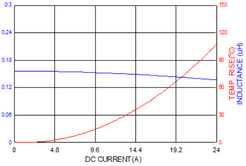
PICQ0612HR15YF
