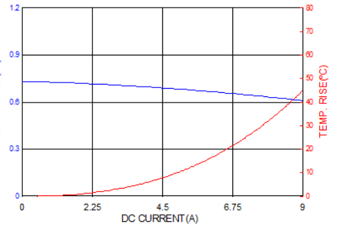
PICQ0612HR68MF
