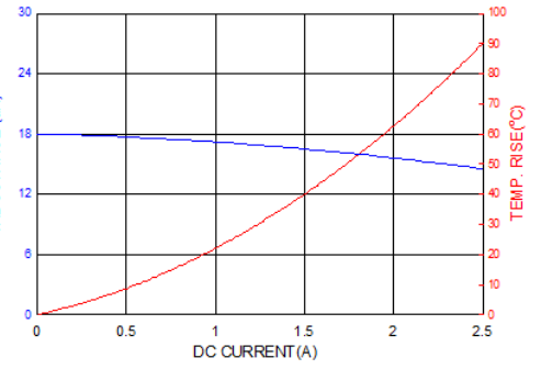
PICQ0612H180MF
