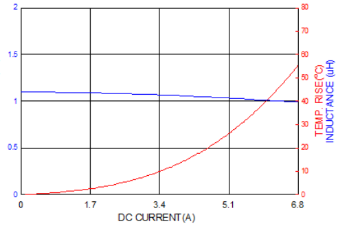
PICQ0612H3R3MF
