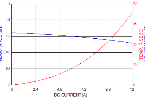
PICQ0503HP1R2MF
