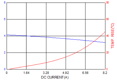
PICQ0503HP4R7MF
