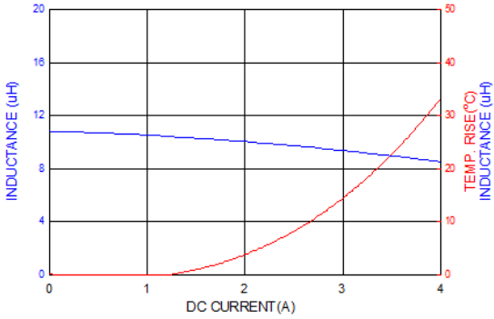
PICQ0503HP100MF
