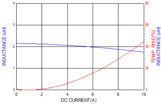
PICQ0503HP2R2MF
