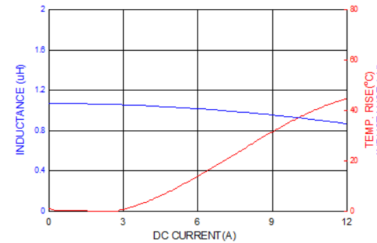
PICQ0503HP1R0MF
