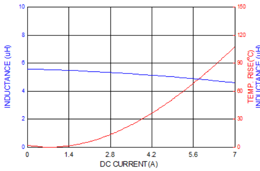
PICQ0503HP5R6MF
