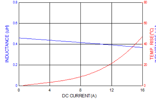
PICQ0503HPR47MF
