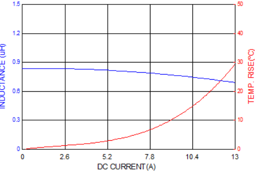
PICQ0503HPR82MF
