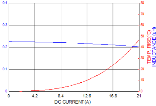
PICQ0503HPR22MF
