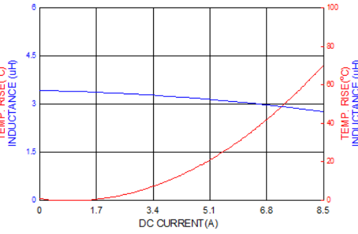
PICQ0503HP3R3MF
