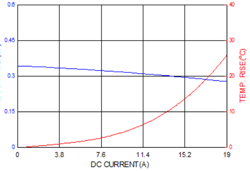
PICQ0503HPR33MF
