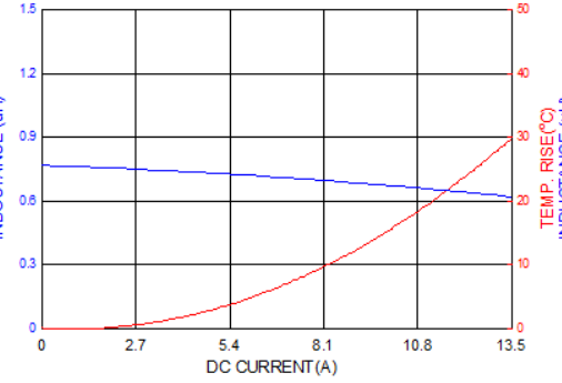
PICQ0503HPR68MF
