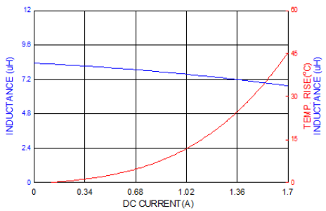
PICQ0312H8R2MF
