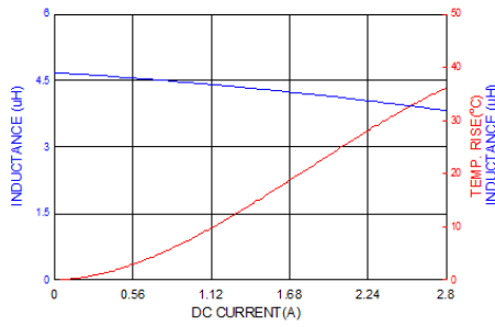
PICQ0312H4R7MF
