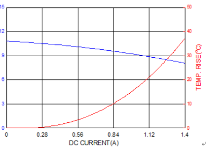
PICQ0312H100MF
